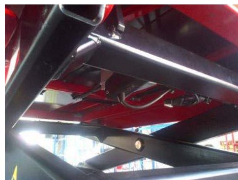
12. Hoeksensor scharen
