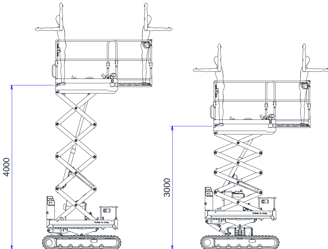
Maximaal toelaatbare transporthoogte (de handmatige nivellering en de regeling van de verplaatsingssnelheid is toegestaan)
