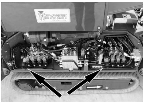
Fig. 140 Knoppen activering proportionele klep wagendeel
