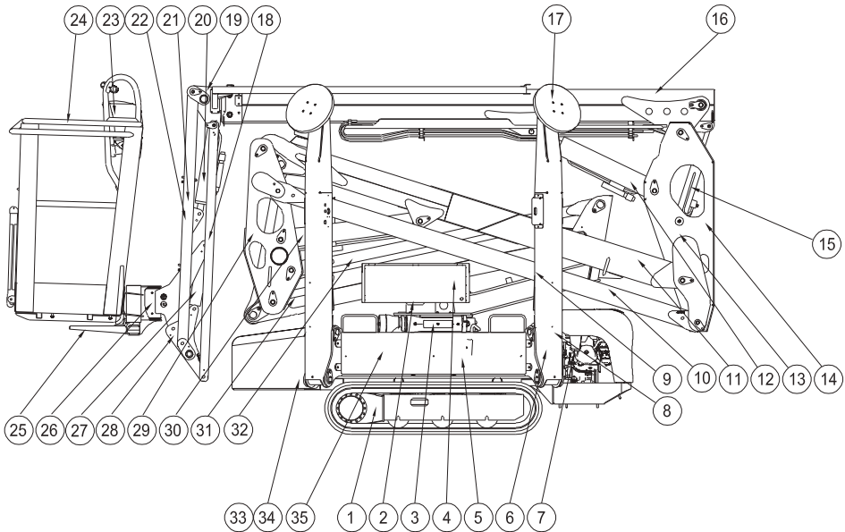
Fig. 5 Begrippen componenten machine
