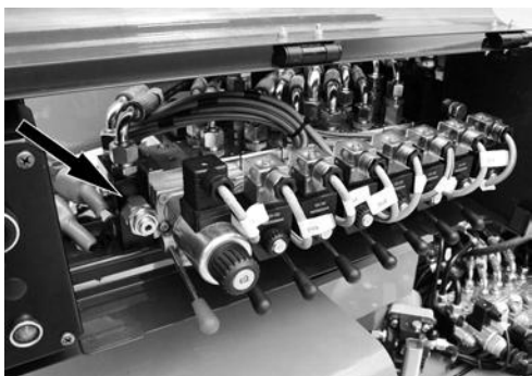
Fig. 8 Overdrukklep hoogwerkerdeel
