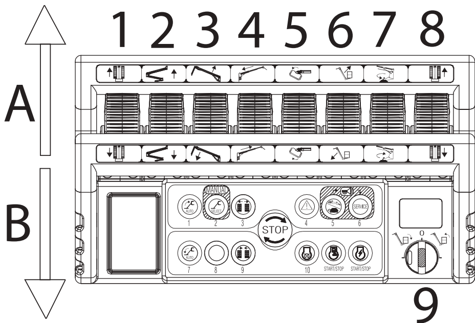
Fig. 49 Bedieningen joysticks
