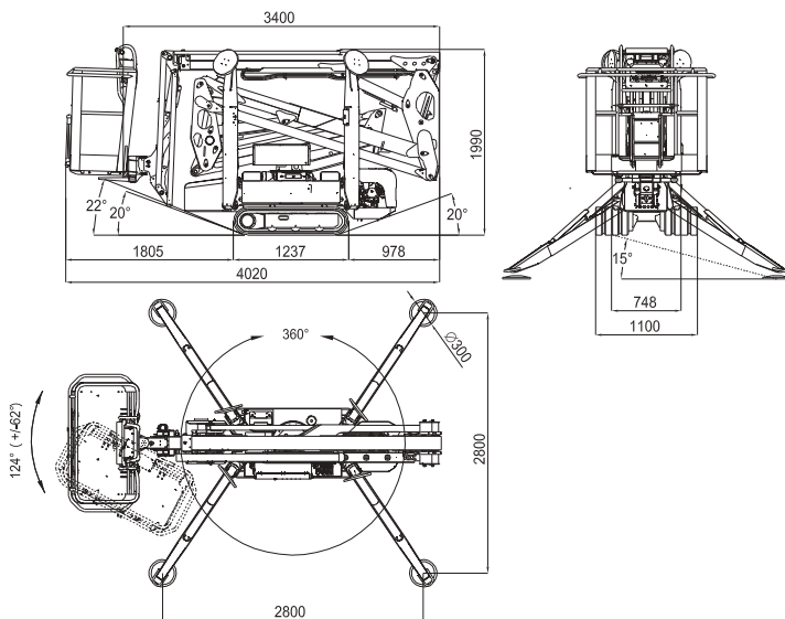
Fig. 4 Standaardversie met tweepersoonsbak
