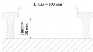
Fig. 171 Profiel oprijplank
