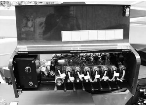
Fig. 125 Bedieningen op verdeler
