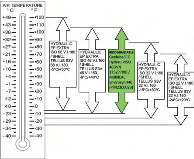
Fig. 149 Gebruikstemperaturen olie
