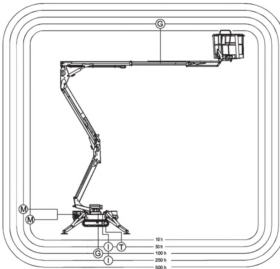
Fig. 151 Schema Smeerpunten
