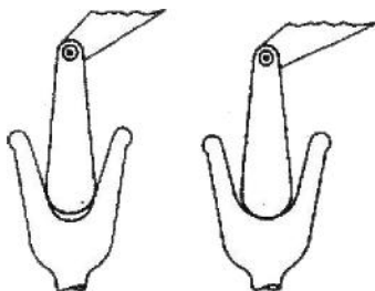
Fig. 186 Voorbeeld verificatie slijtage poelies
