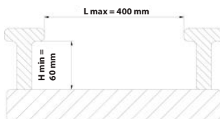
Fig. 194 Profiel oprijplank
