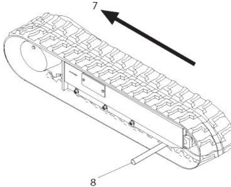
Fig. 179 Voorbeeld montage rupsband
