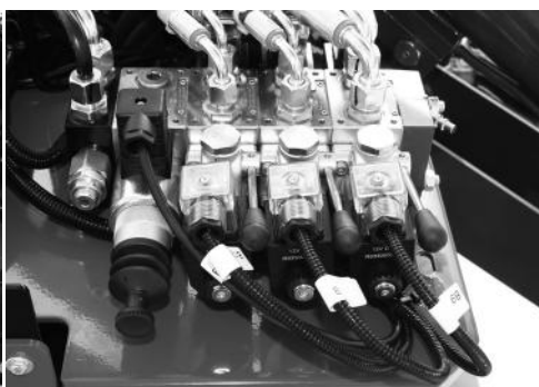
Fig. 93 Bedieningen op verdeler rechts
