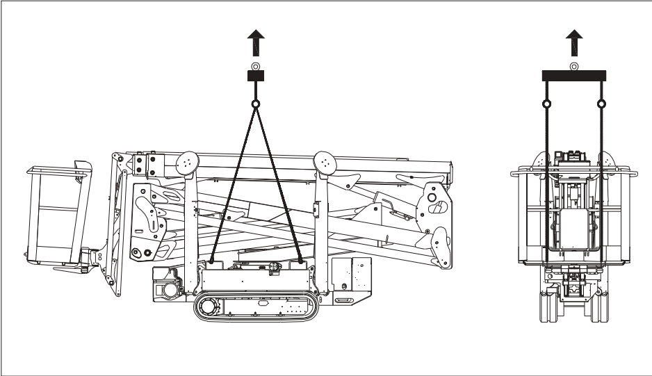
Fig. 197 Hijsschema met kabels of kettingen
