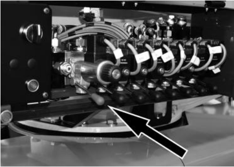
Fig. 140 Knop activering proportionele klep hoogwerkerdeel
