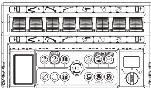
Fig. 122 Afstandsbediening
