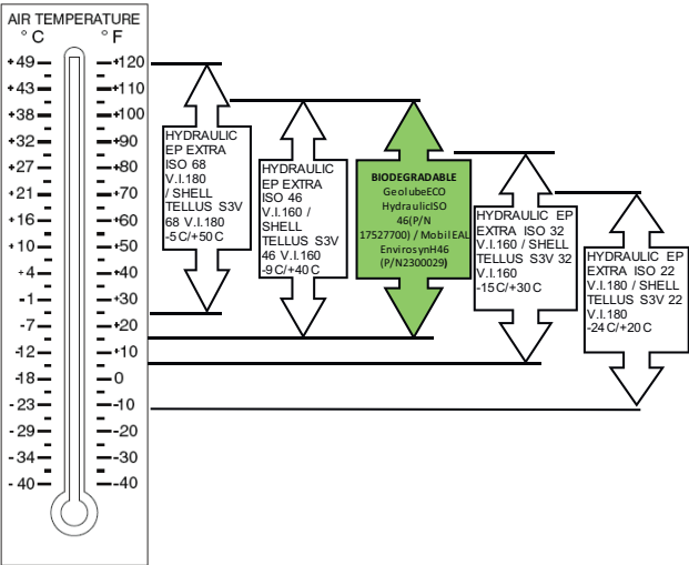
Fig. 165 Gebruikstemperaturen olie
