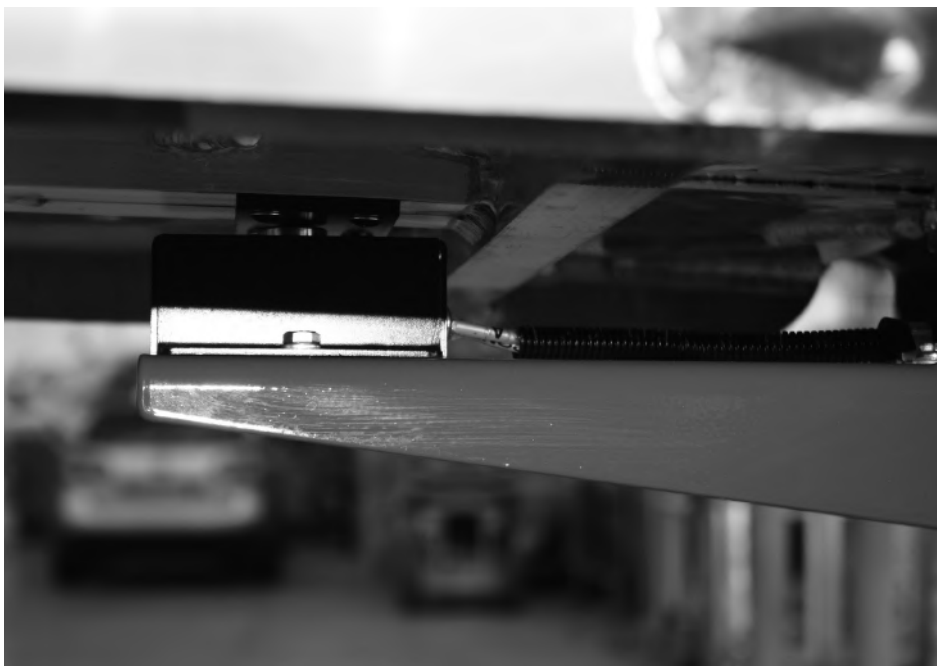
Fig. 20 Laadsensor
