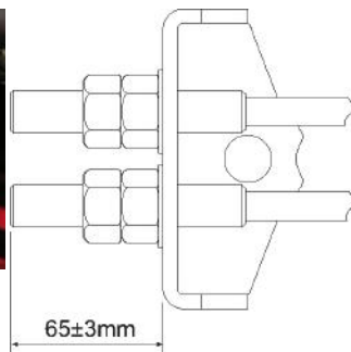
Fig. 190 Bijv. Spanning Aanpassing kabels
