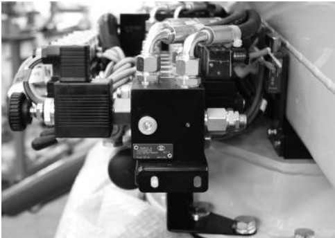
Fig. 8 Overdrukklep bovenbouw
