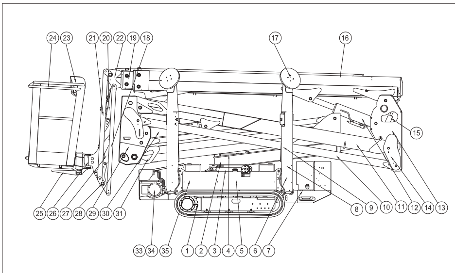
Fig. 5 Begrippen componenten machine
