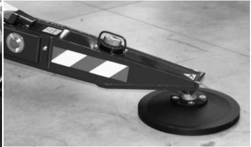
Fig. 110 Controlelampje stempel op de grond
