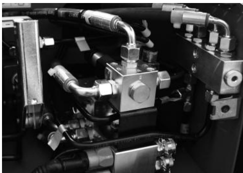
Fig. 154 Omschakelaar luchtdeel - wagendeel
