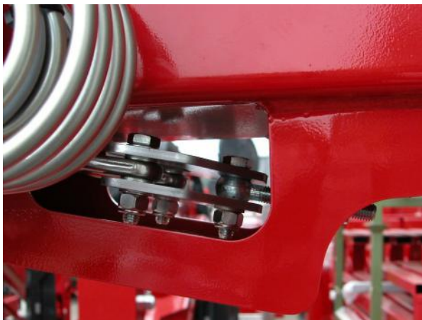
Fig. 187 Balansjuk bevestiging terugvoerkabels
