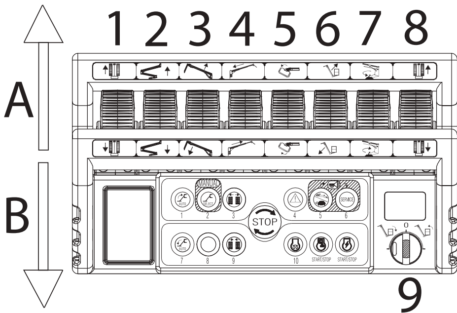
Fig. 64 Bedieningen joysticks
