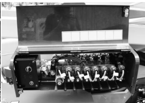
Fig. 73 Hydraulische bedieningen aan de grond
