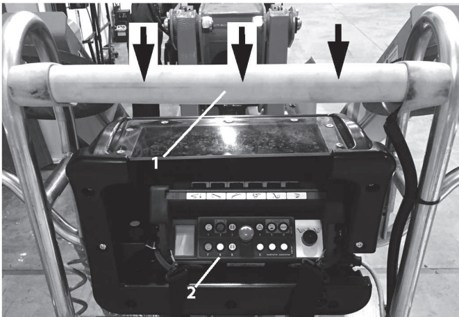
Fig. 75 1-Sensor SkyGuard™ 2- SkyGuard™ By-pass (knop nummer 8)
