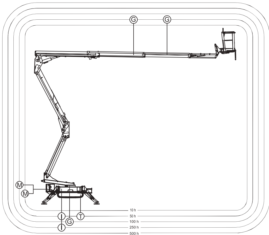
Fig. 167 Schema Smeerpunten
