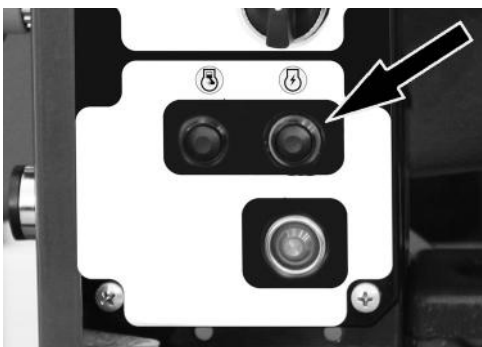
Fig. 86 Startknop elektromotor
