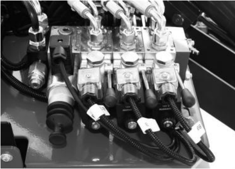
Fig. 157 Voorbeeld bedieningen op verdeler
