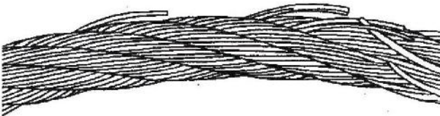
Fig. 184 Voorbeeld gebroken draden
